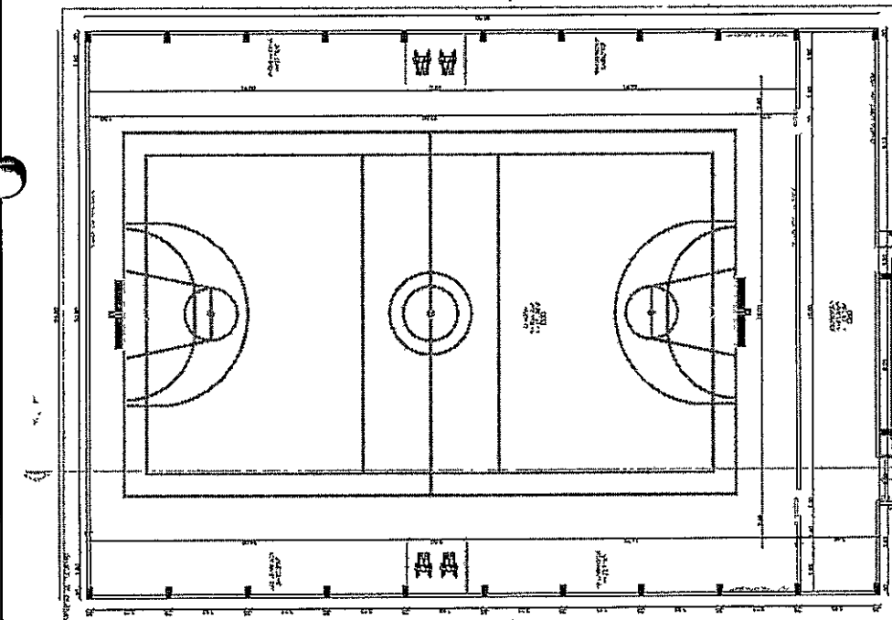
PLANTA BAIXA
